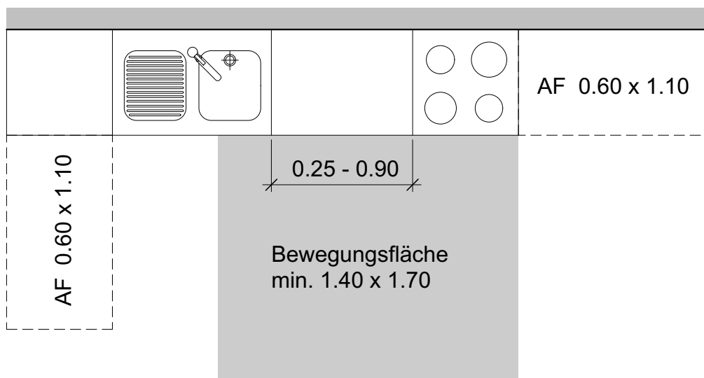
Beispiel Einfrontenküche
