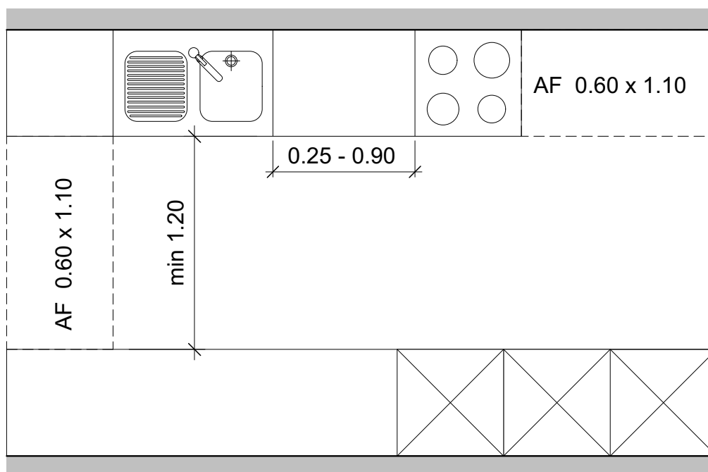
Beispiel Zweifrontenküche
